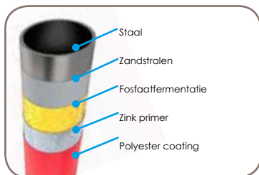
Bescherming tegen roest dankzij verzinkt staal met poedercoating
